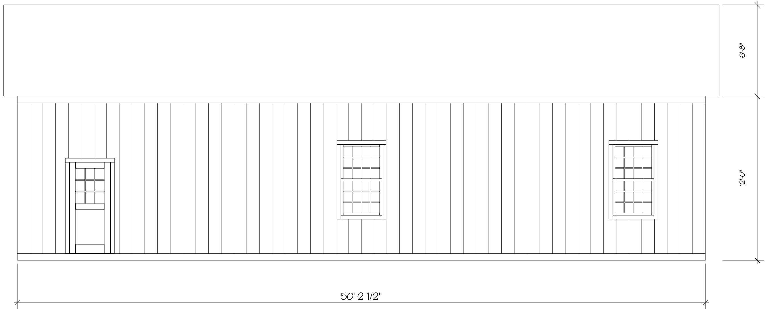
4 Side Elevation Scale: 1/4" = 1'-0"
